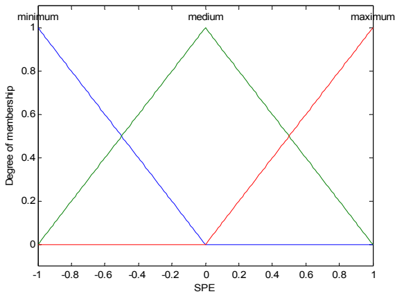
Fig. 9a: Membership function of SPE
