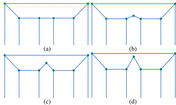
Fig. 1: Transformer core type (a) T-joint 90^\circ , (b) T-joint 23^\circ , (c) T-joint 45^\circ and (d) T-joint 60^\circ
